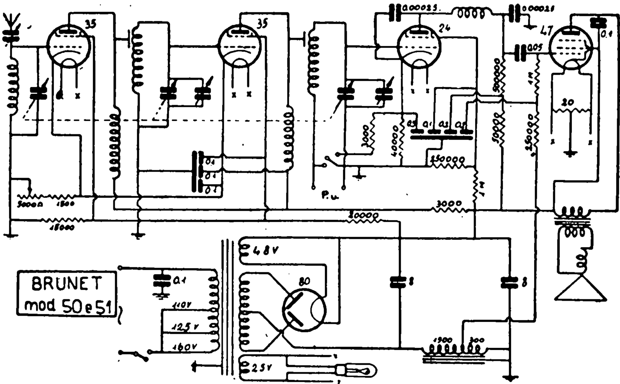
BRUNET Soc. An. — Modelli 50 e 51. - (Le valvole '35 possono venir sostituite con '51, la '24 con la '57). Produzione 1932.
